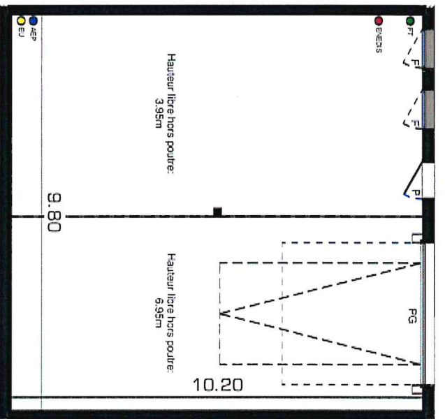
PLAN RDC
